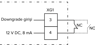
Şek. 13: Prensiyel devre şeması: Harici bir şalter kontağının bağlanması (standart ayar: NC)
