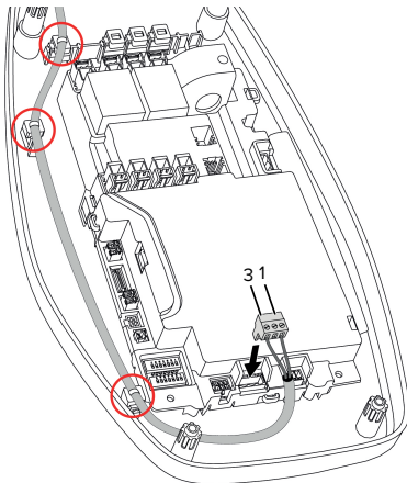
Abb. 9: Anschluss Arbeitsstromauslöser
