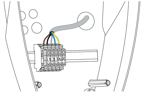
Ilustr. 8: Przyłącze zasilania napięciowego
