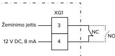
Pav. 13: Principinė sujungimo schema: išorinio jungimo kontakto jungties prijungimas (standartinis nustatymas: NC)
