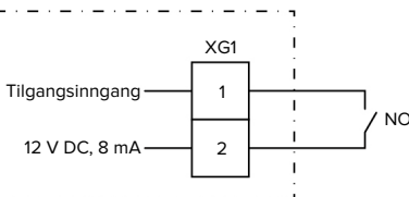
Fig. 15: Prinsipielt koblingsskjema: Tilgangsinngang
