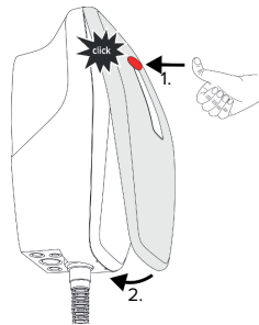
Afb. 18: Frontcover aanbrengen - 1
