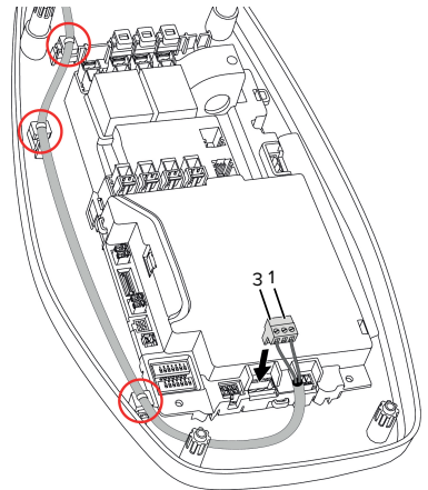
Fig. 9 : Raccordement du limiteur de courant de travail
