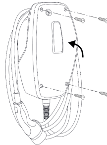
Fig. 16: Chiusura del prodotto
