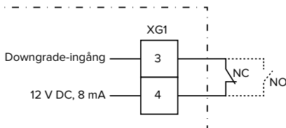
Fig. 13: Principkopplingschema: Anslutning av en extern brytarkontakt (standardinställning: NC)
