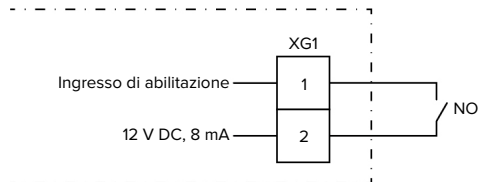
Fig. 15: Schema di principio: Ingresso di abilitazione
