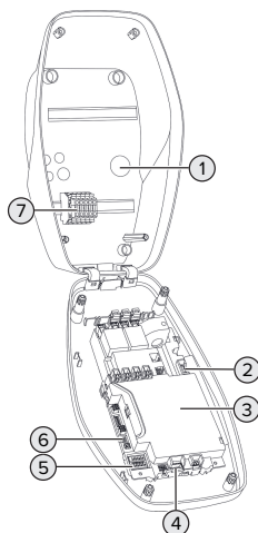
Fig. 3: Vy inifrån
