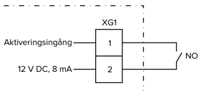
Fig. 15: Principkopplingschema: Aktiveringsingång
