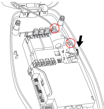
Abb. 12: Anschluss Downgrade-Eingang
