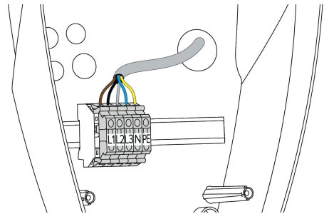
Fig. 8: Anslutning matarspänning
