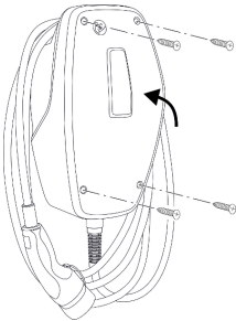
Kuva 16: Tuotteen sulkeminen
