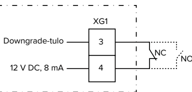
Kuva 13: Periaatekytkentäkaavio: ulkoisen kytkentäkontaktin liitäntä (vakioasetus: NC)
