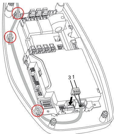
Obr. 9: Přípojka vypínače pracovního proudu
