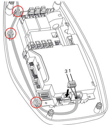
Afb. 9: Aansluiting arbeidsstroomactiveringsschakelaar
