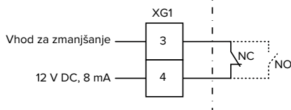
sl. 13: Osnovna vezalna shema: Priključitev zunanega preklopnega kontakta (standardna nastavev: NC)
