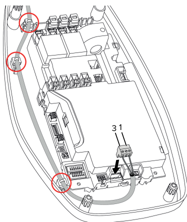
Fig. 9: Anslutning arbetsströmutlösare
