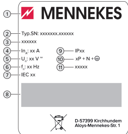
Fig. 1: Produkt-typskylt (mall)
