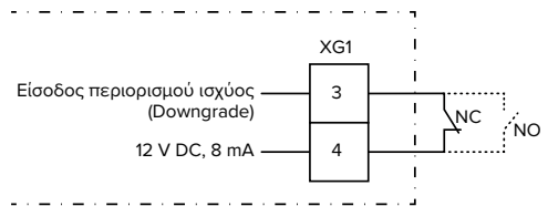
Εικ. 13: Διάγραμμα συνδεσμολογίας: Σύνδεση εξωτερικής επαφής μεταγωγής (βασική ρύθμιση: NC)
