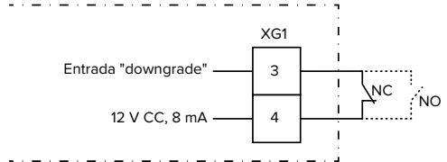
Fig. 13: Esquema de princípio: ligação de um contacto de comutação externo (configuração padrão: NF)
