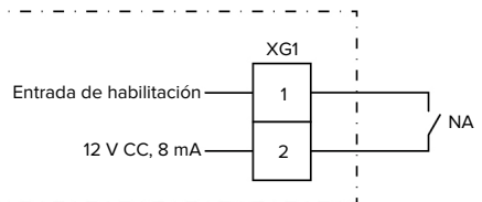
Fig. 15: Esquema de principio: Entrada de habilitación
