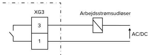
Fig. 10: Principskema: Tilkobning af en ekstern arbejdsstrømsudløser
