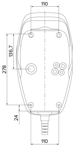
Fig. 6: Boredimensjoner [mm]
