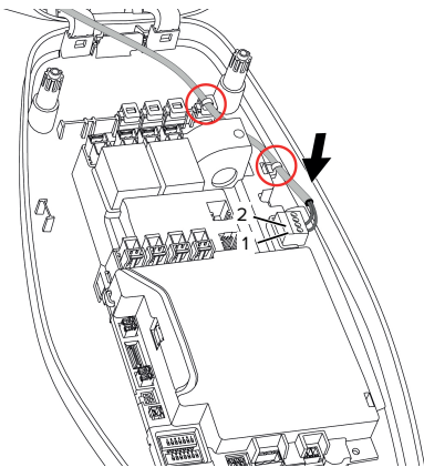
Abb. 14: Anschluss Freigabe-Eingang
