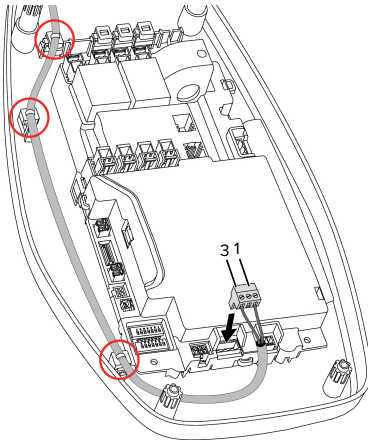
Kuva 9: Työvirtalaukaisijan liitäntä
