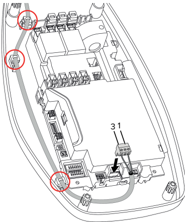
Fig. 9: Collegamento sganciatore di apertura
