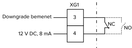
13. Ábra: Elvi kapcsolási rajz: Külső kapcsolóérintkező csatlakoztatása (normál beállítás: NC)
