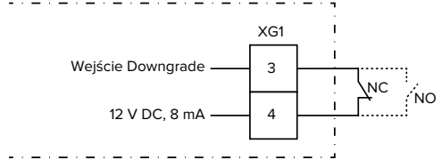
Ilustr. 13: Schemat blokowy: podłączenie zewnętrznego styku przełączającego (ustawienie standardowe: NC)
