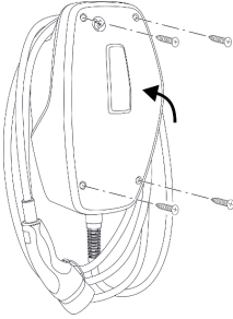
Şek. 16: Ürünün kapatılması
