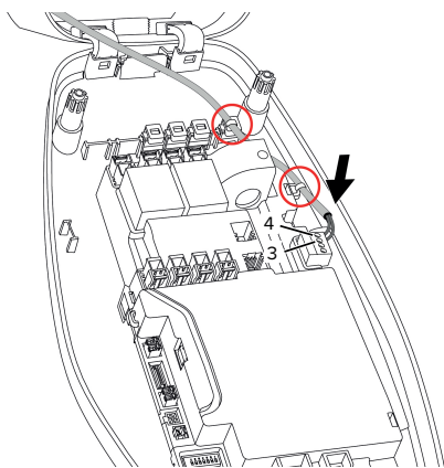
Fig. 12: Tilslutning downgrade-indgang
