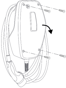
Şek. 5: Ürünün açılması
