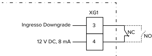
Fig. 13: Schema di principio: collegamento di un contatto di commutazione esterno (impostazione di default: NC)
