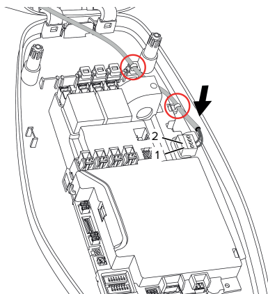
Ilustr. 14: Zaciski przyłączeniowe – wejście zwalniające
