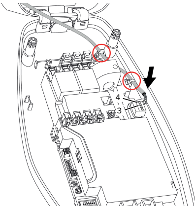
Kuva 12: Downgrade-tulon liitäntä
