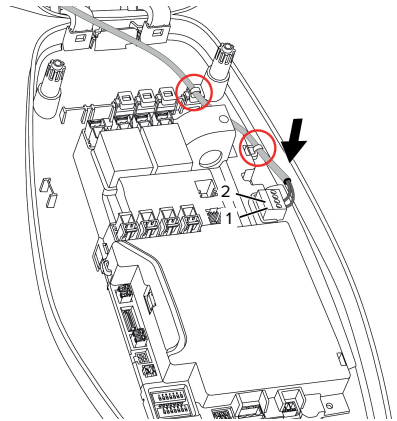
Fig. 14 : Raccordement de l'entrée de validation
