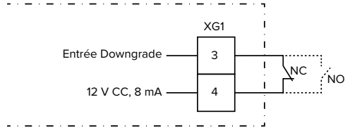
Fig. 13 : Schéma de principe : raccordement d'un contact électrique externe (réglage par défaut : NF)
