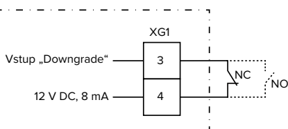
Obr. 13: Základní schéma zapojení: Připojení externího spínacího kontaktu (standardní nastavení: NC)
