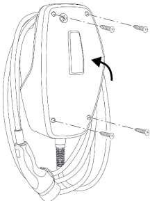
16. Ábra: A termék lezárása
