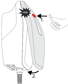
Ilustr. 18: Zakładanie pokrywy przedniej - 1
