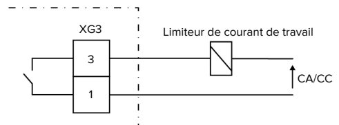
Fig. 10 : Schéma de principe : Raccordement d'un limiteur de courant de travail externe
