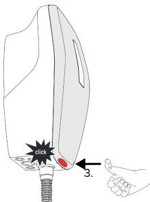
Fig. 19 : Monter le cache frontal - 2
