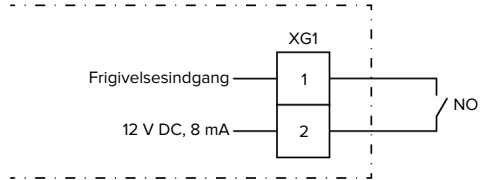
Fig. 15: Principskema: Frigivelsesindgang
