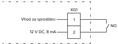
sl. 15: Osnovna vezalna shema: Vhod za sprostitve
