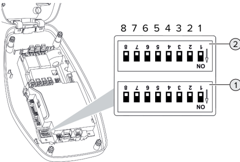
Afb. 11: Dipschakelaar (uitleveringstoestand)
