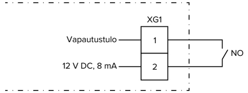
Kuva 15: PeriaatekytKentäkaavio: vapautustulo
