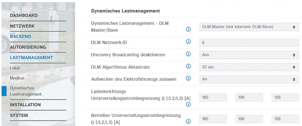
Abb. 23: Weboberfläche des DLM-Masters zur Konfiguration von Lastmanagement
