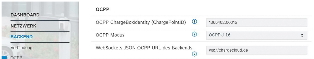
Abb. 15: Weboberfläche von jeder vernetzten Ladestation zur Konfiguration des OCPP Kommunikationsprotokolls
