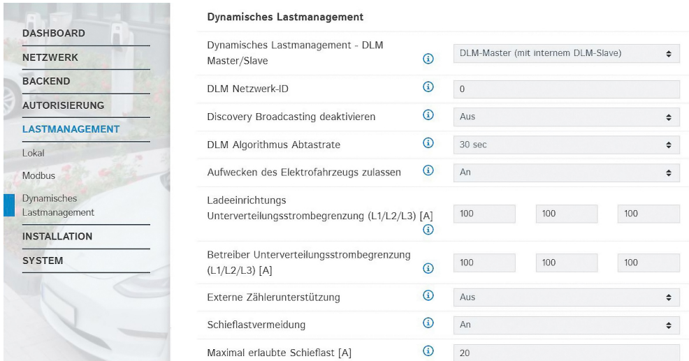
Abb. 33: Weboberfläche des DLM-Masters zur Konfiguration von Schiefastvermeidung
