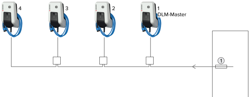
Abb. 21: Lastmanagement bei einem Parkplatz mit mehreren Ladepunkten (Beispiel: Produkte mit integrierten Fehlerstromschutzschalter und Leitungsschutzschalter)
