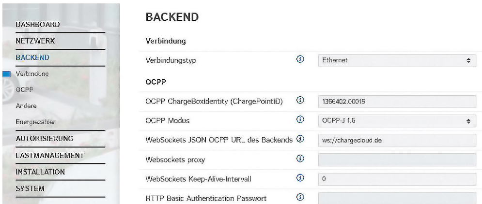
Abb. 19: Weboberfläche zur Anbindung mehrere Ladepunkte an ein Backend-System über LAN / Ethernet (RJ45) und einen externen Router
