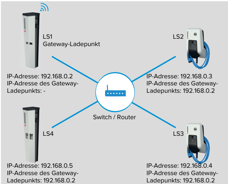
Abb. 16: LS1 als Gateway-Ladepunkt
