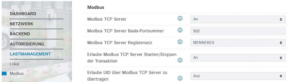
Abb. 30: Weboberfläche zur Konfiguration von Modbus TCP
